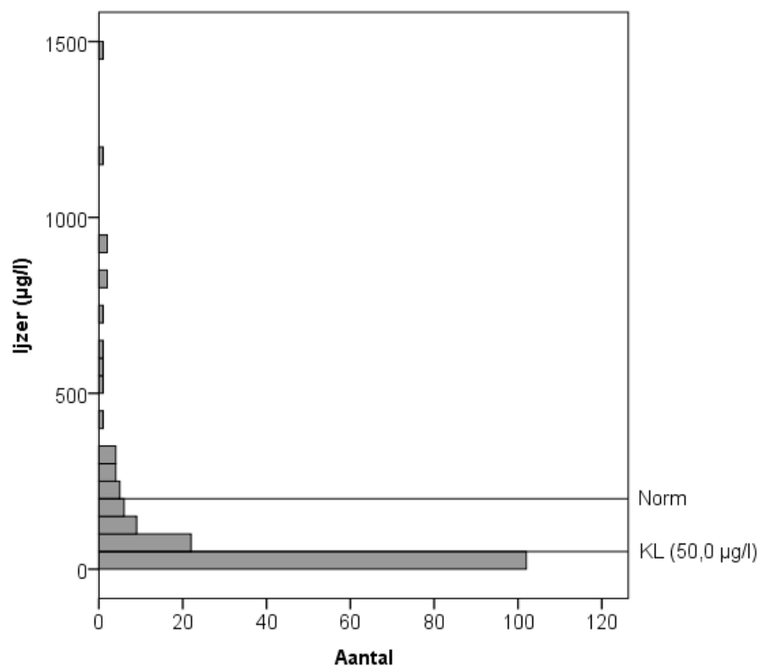
Figuur 9 Histogram voor ijzergehalte in putwaterstalen. Nota: KL=Kwantificatielimiet; mediaan onder KL; 8 waarden buiten de figuur (3820, 4350, 4980, 5370, 7420, 8050, 13500 \mu\text{g/l} ).
