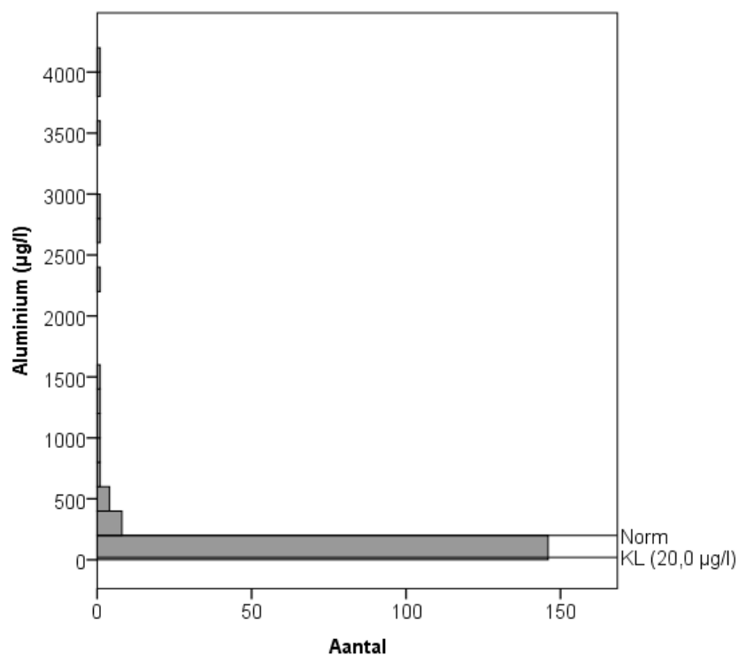
Figuur 10 Histogram voor aluminiumgehalte in putwaterstalen. Nota: KL=Kwantificatielimiet; mediaan onder KL; 2 waarden buiten de figuur (5990, 7410 \mu\text{g/l} ).
